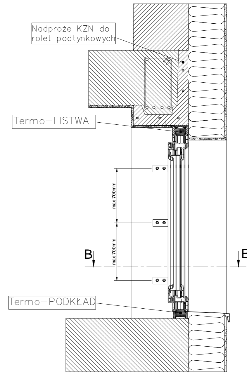
Rozwiązanie dla drzwi Termo-Listwa; Termo-Parapet
