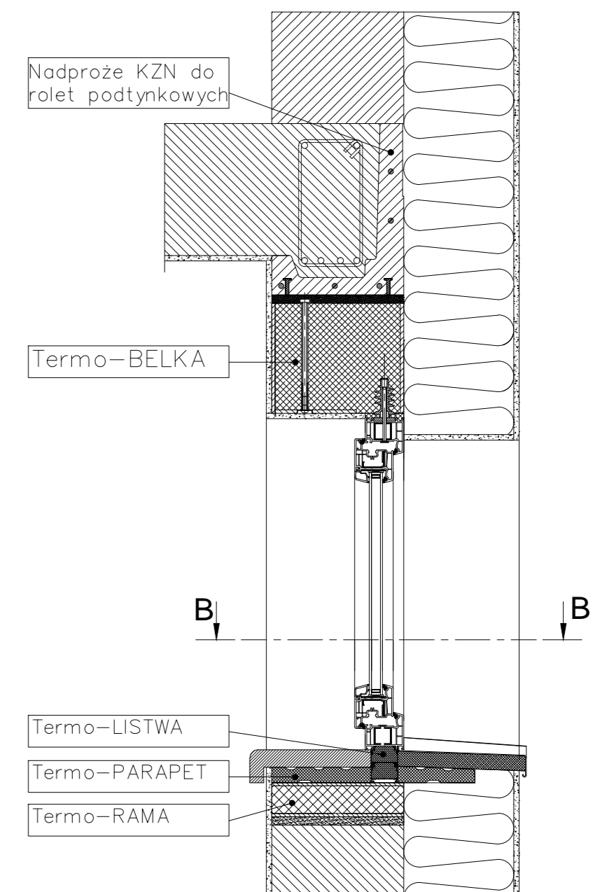
Rozwiązanie Termo-Listwa; Termo-Parapet; Termo-BELKA; Termo-RAMA montaż w świetle muru
