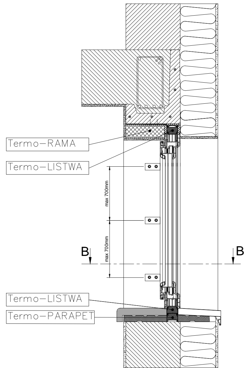
Rozwiązanie Termo-Listwa; Termo-Parapet
